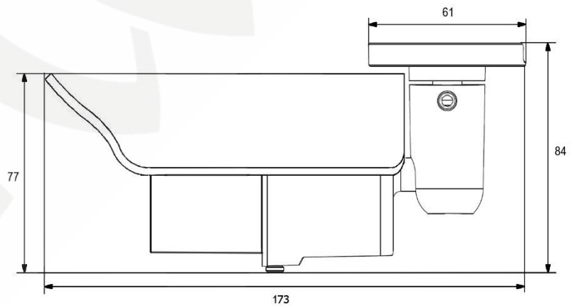
BD4640RC(V)
